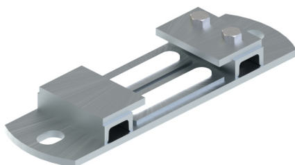
Typ 302-121-U-SH Abb. Gr. 5
