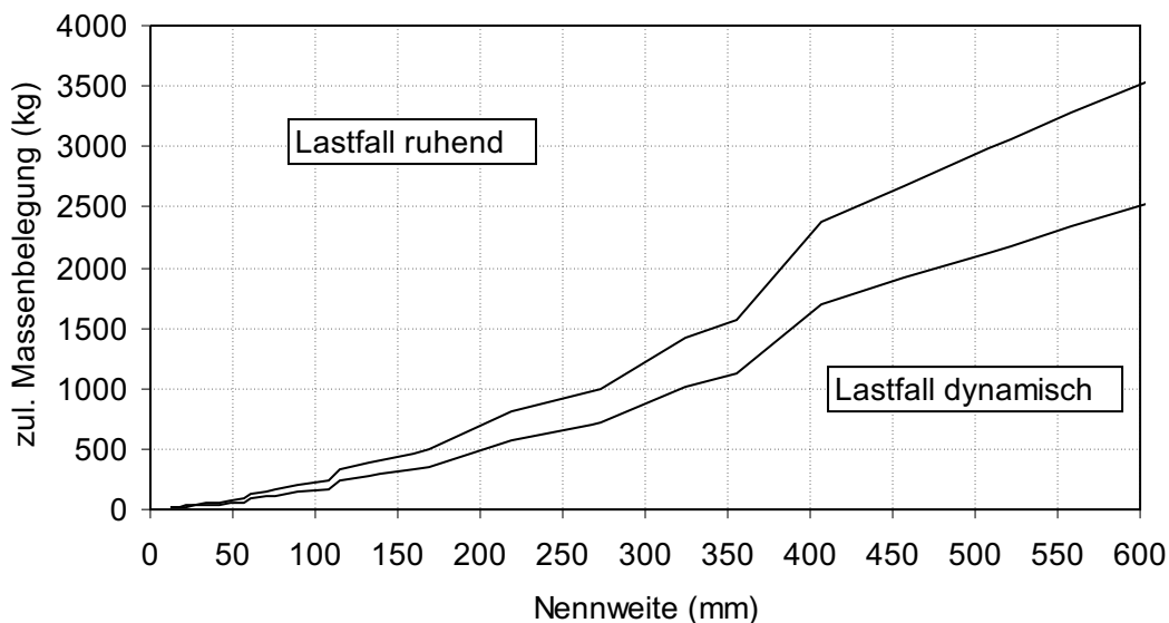
Zul. Massenbelegung für dipa Typ 170 (2 Punkt Aufhängung)
