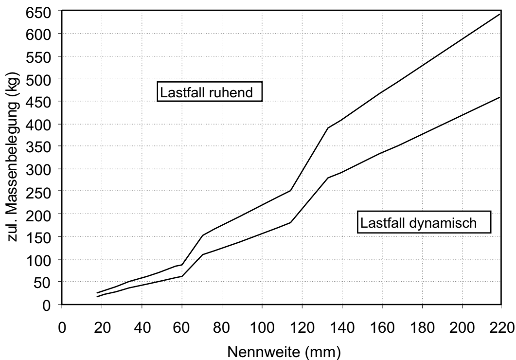
Zul. Massenbelegung für dipa Typ 175
