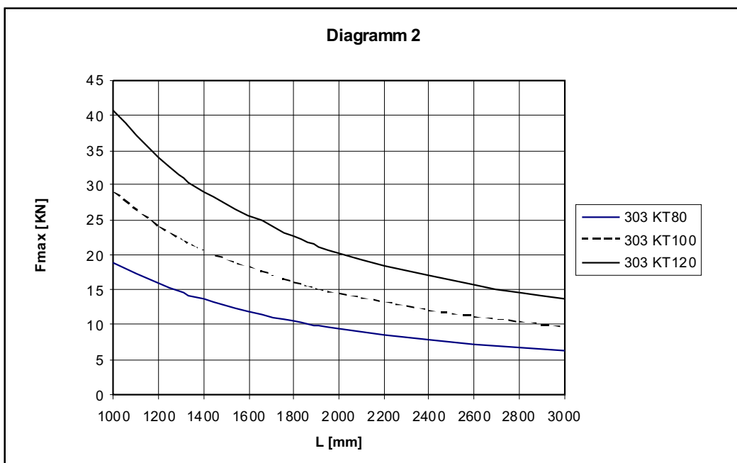
Diagramm 2 : Punktbelastung (Mitte) für freistehende Brücke bei statischer Last
