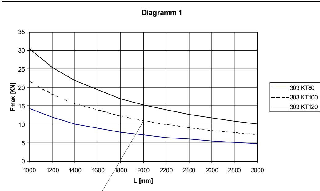
Diagramm 1 : Punktbelastung (Mitte) für Winkelkonsole bei statischer Last
